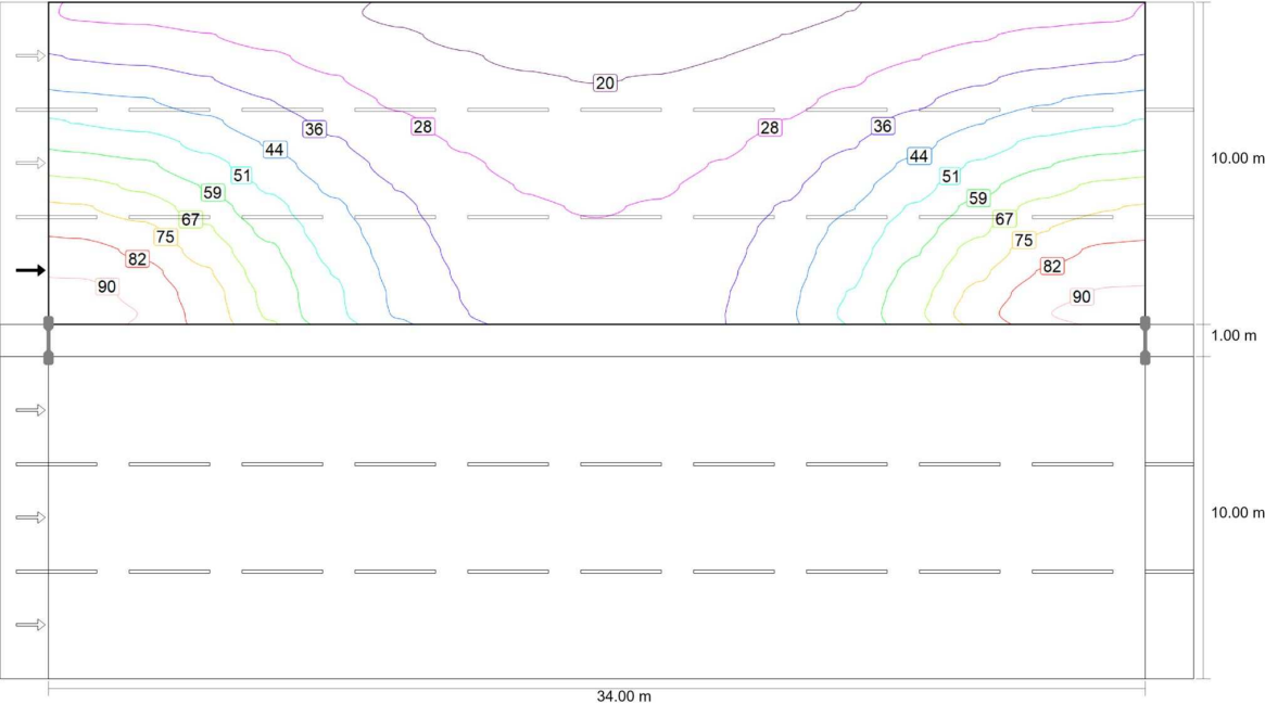
Valor de manutenção de iluminância horizontal [lx] (Linhas de isolux)
