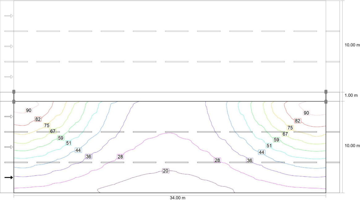
Valor de manutenção de iluminação horizontal [lx] (Linhas de isolux)
