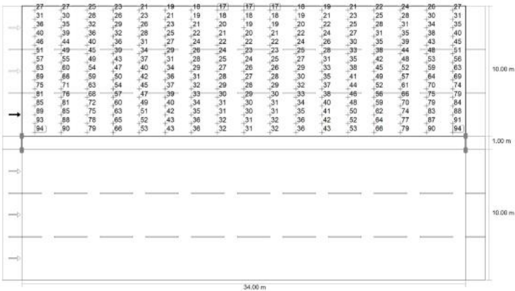
Valor de manutenção de iluminação horizontal [lx] (Grelha de valores)
