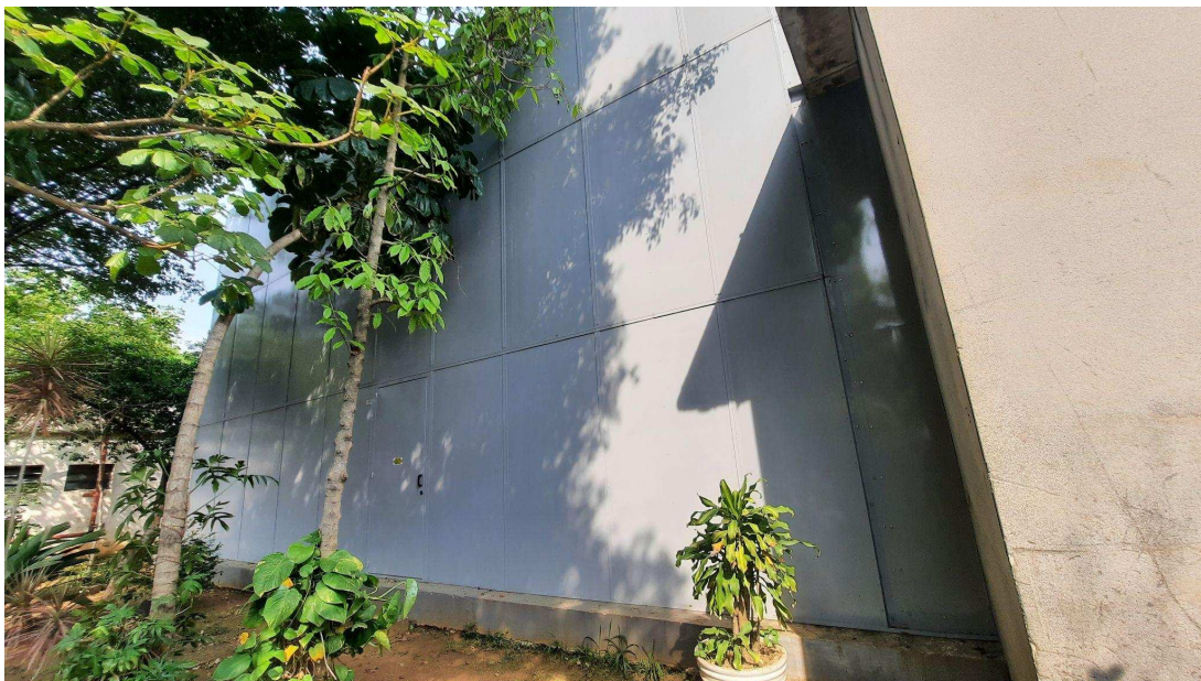
Figura 3 - Proteção acústica lado externo. Fonte: Foto in loco.
