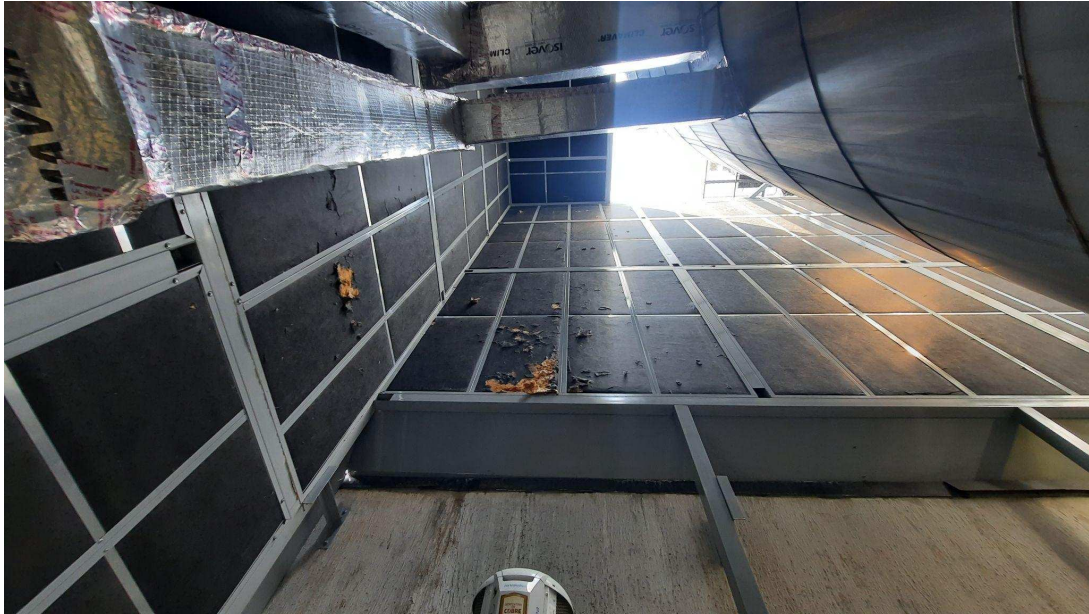
Figura 2 - Proteção acústica lado interno. Fonte: Foto in loco.
