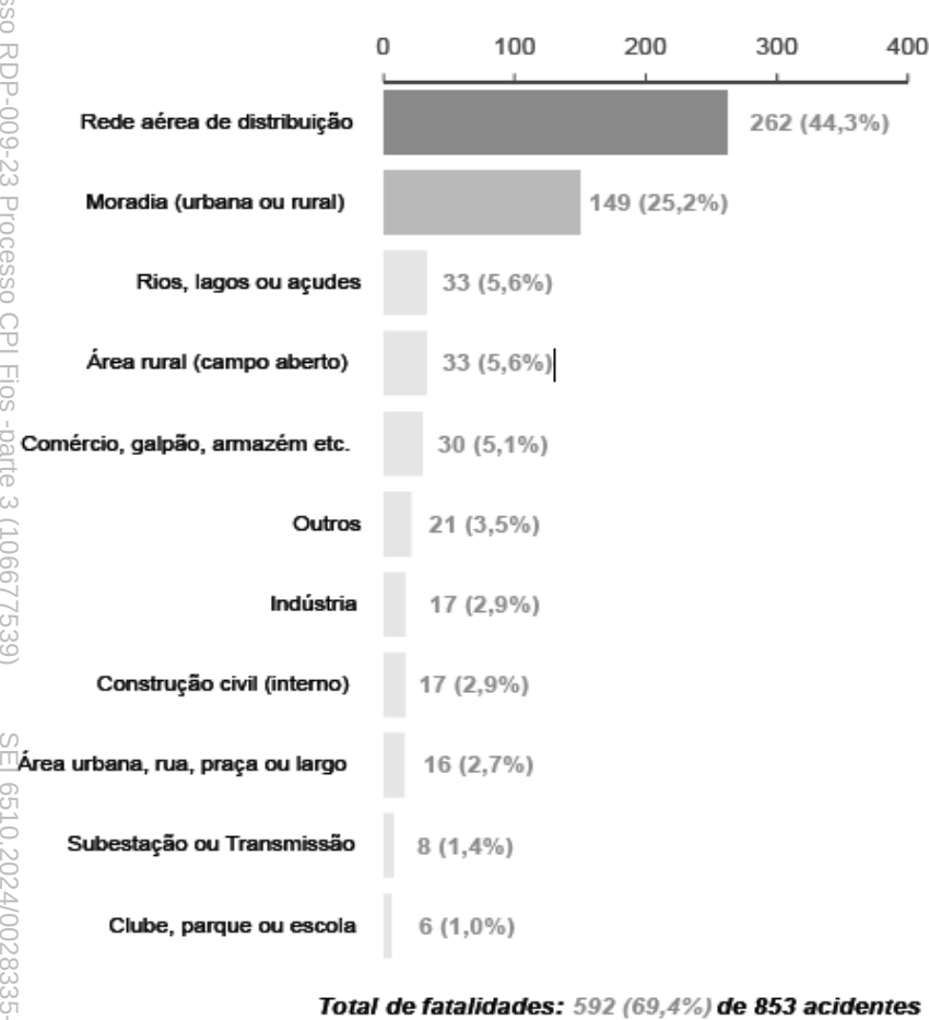
Gráfico 14 - Mortes por choque elétrico por local de ocorrência 2022
