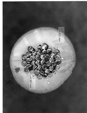
Figura 9 Cabo Comum (2,5mm 2 ) com 40 fios internos de cobre e um diâmetro total de 3,6mm
