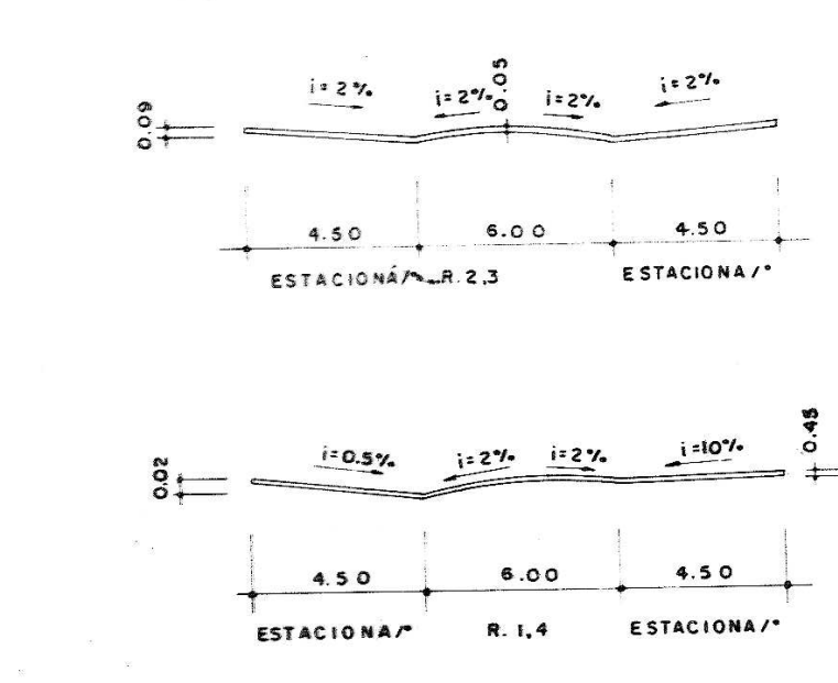
SEÇÃO DO ESTACIONAMENTO ESCALA 1:200
