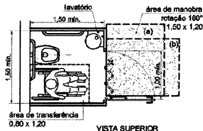
Figura 126 — Boxe para bacia sanitária — Reformas — Área de manobra externa — Exemplo
