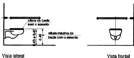
Figura 119 — Adequação de altura da bacia sanitária suspensa
