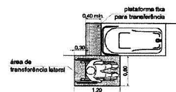
Figura 131 — Plataforma fixa para transferência
