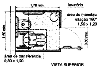
Figura 125 — Boxe para bacia sanitária - Transferência lateral - Exemplo
