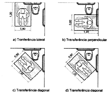
Figura 114 — Áreas de transferência para bacia sanitária
