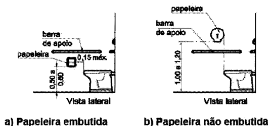
Figura 143 — Figura 31 — Papeleiras
