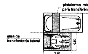
Figura 132 — Plataforma para transferência móvel
