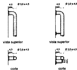
Figura 113 — Barras de apoio
