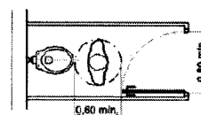
Figura 123 — Boxe com porta abrindo para o interior
