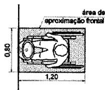
Figura 139 — Área de aproximação para P.C.R.
