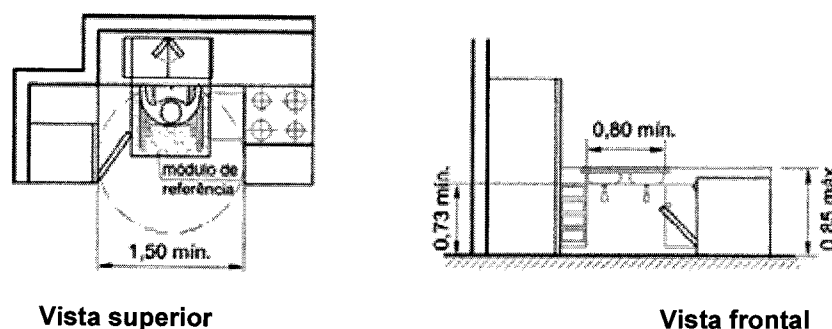
Figura 154 — Cozinha — Exemplo
