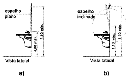
Figura 142 — Acessórios sanitários — Espelhos
