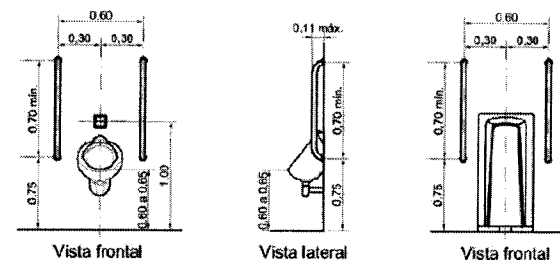
Figura 140 — Mictórios — Exemplos
