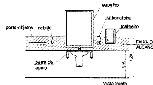
Figura 141 — Acessórios junto ao lavatório — Exemplo
