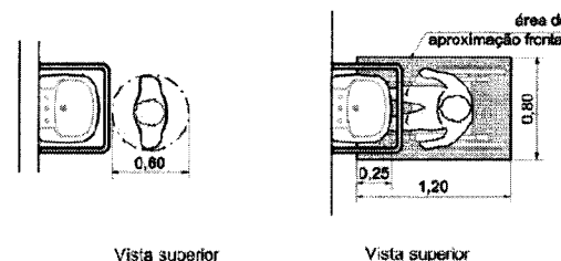
Figura 134 — Área de aproximação para P.M.R.
