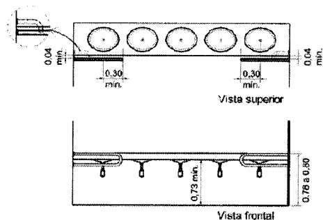
Figura 137 — Lavatórios embutidos em bancadas — Exemplo
