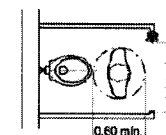
Figura 124 — Boxe com porta sanfonada
