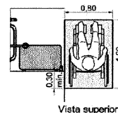
Figura 127 — Área de transferência para box de chuveiro — Exemplo
