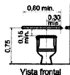
Figura 118 — Bacia sanitária com caixa acoplada
