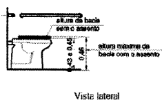
Figura 120 — Adequação de altura da bacia sanitária alongada
