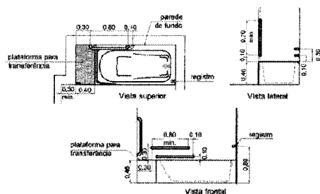
Figura 133 — Banheira — Exemplo
