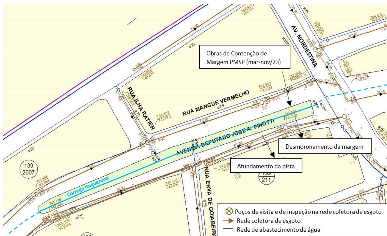
Imagem 01: Av Deputado José Aristodemo Pinotti - Tela do SIGNOS adaptada com redes de Água e Esgoto, com indicação das obras da Prefeitura Municipal de São Paulo – PMSP.
