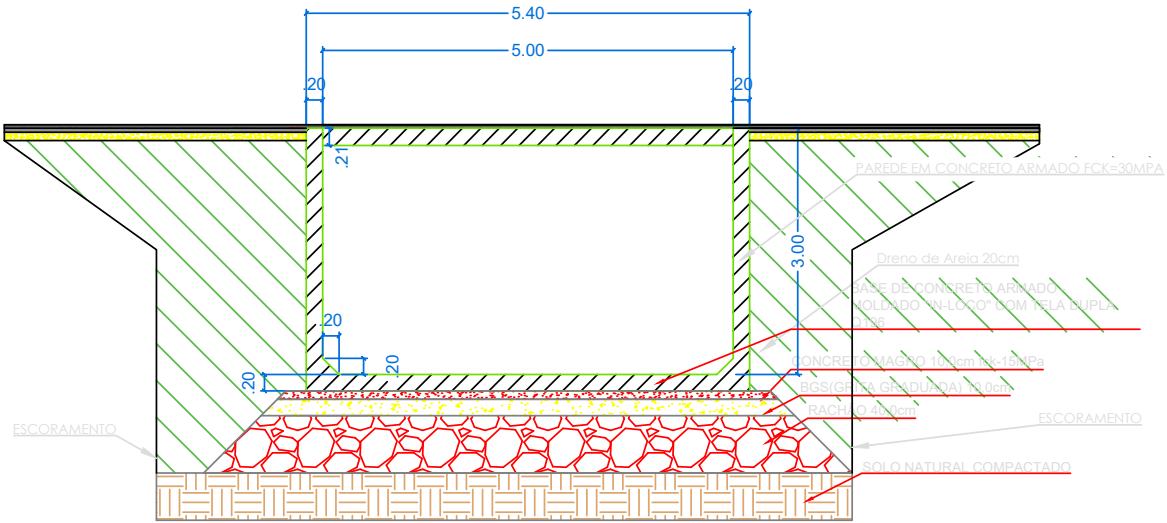
CORTE GALERIA FECHADA ESCALA 1:100
