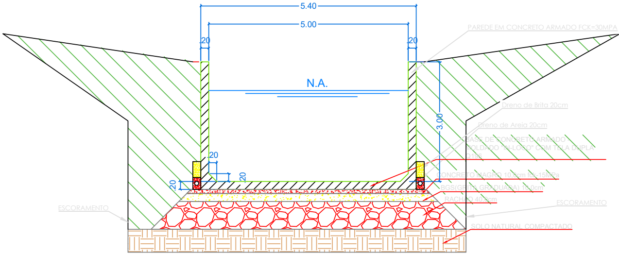
CORTE GALERIA ABERTA ESCALA 1:100
