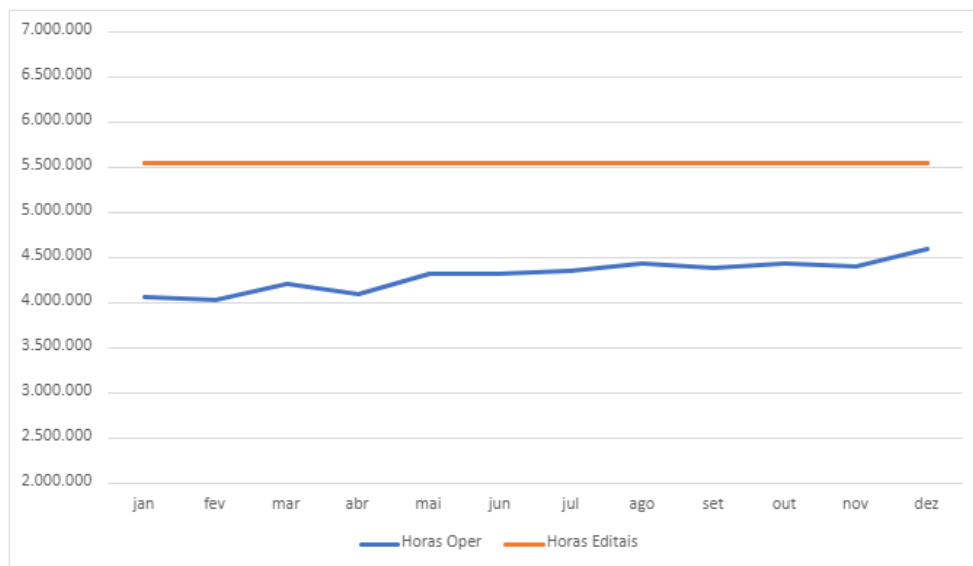
Gráfico 10 – Comparativo entre horas operadas totais e horas edital (%)
