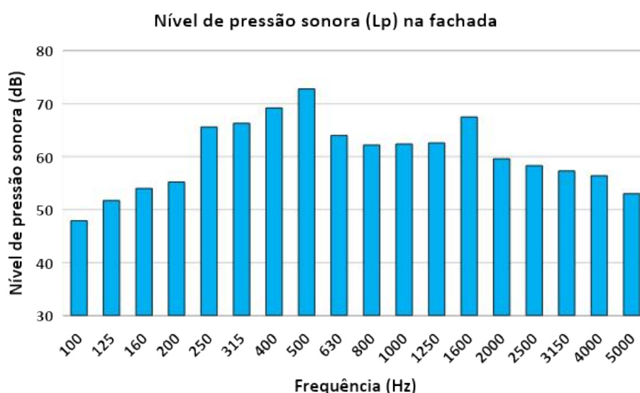
Figura 6: Nível de Pressão Sonora – Ar condicionado
