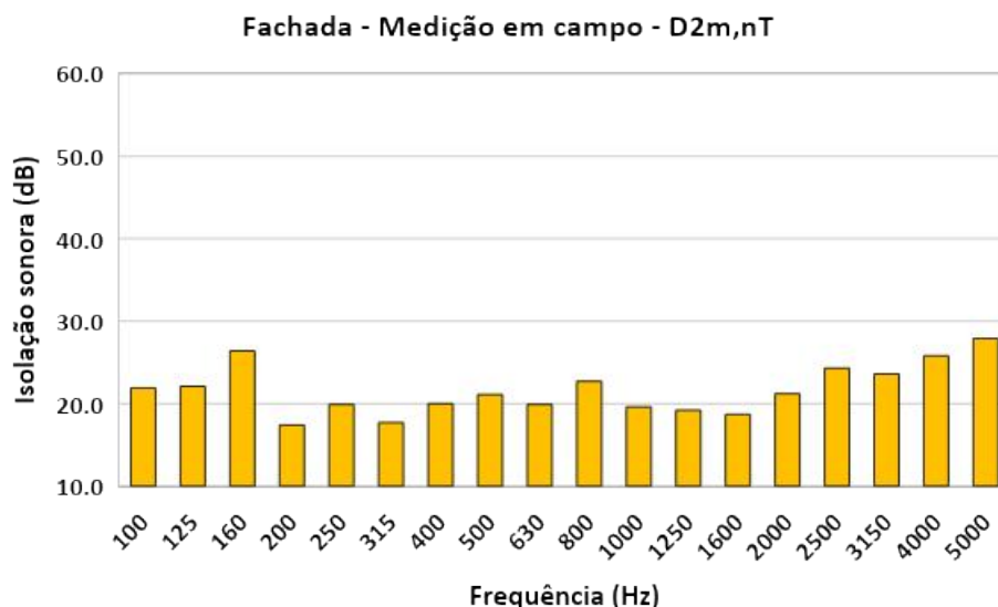
Figura 4: Isolamento sonora de fachada, casa térrea
