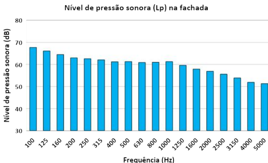
Figura 8: Nível de Pressão Sonora – Tráfego de veículos
