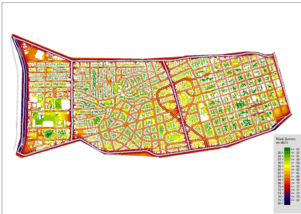
Figura 1 – Exemplo de mapa de ruído elaborado pelo IPT
