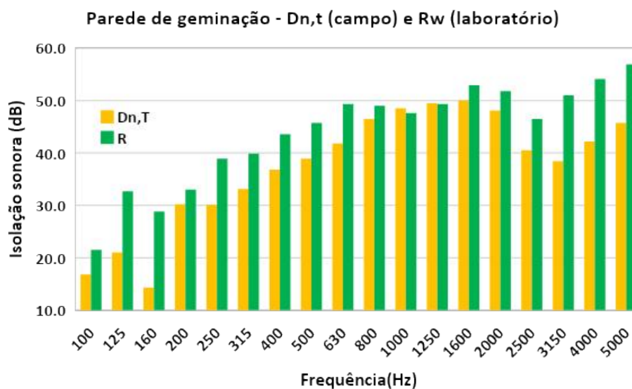
Figura 3: Isolação sonora de parede divisória entre unidades
