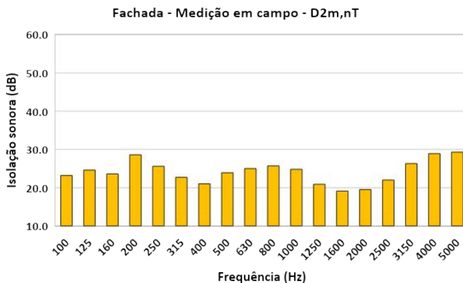
Figura 5: Isolamento sonora de fachada, apartamento
