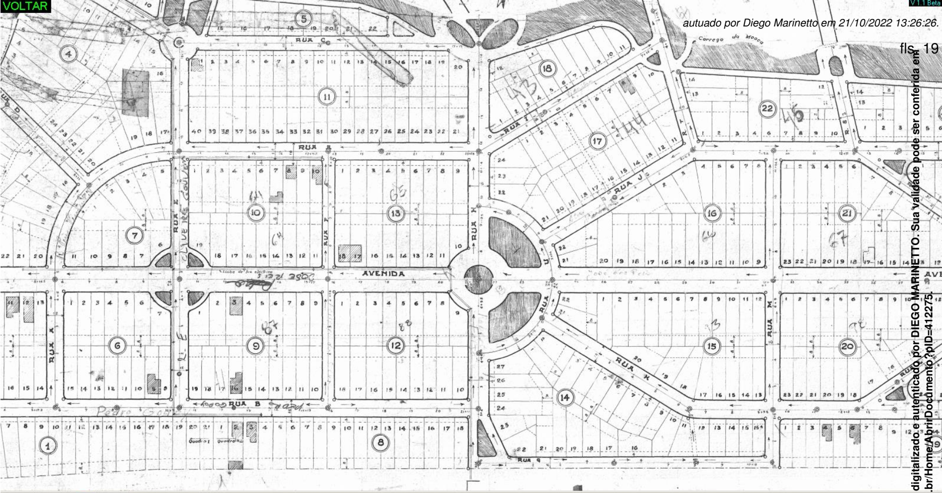
Planta (parcial) ARR 0026
