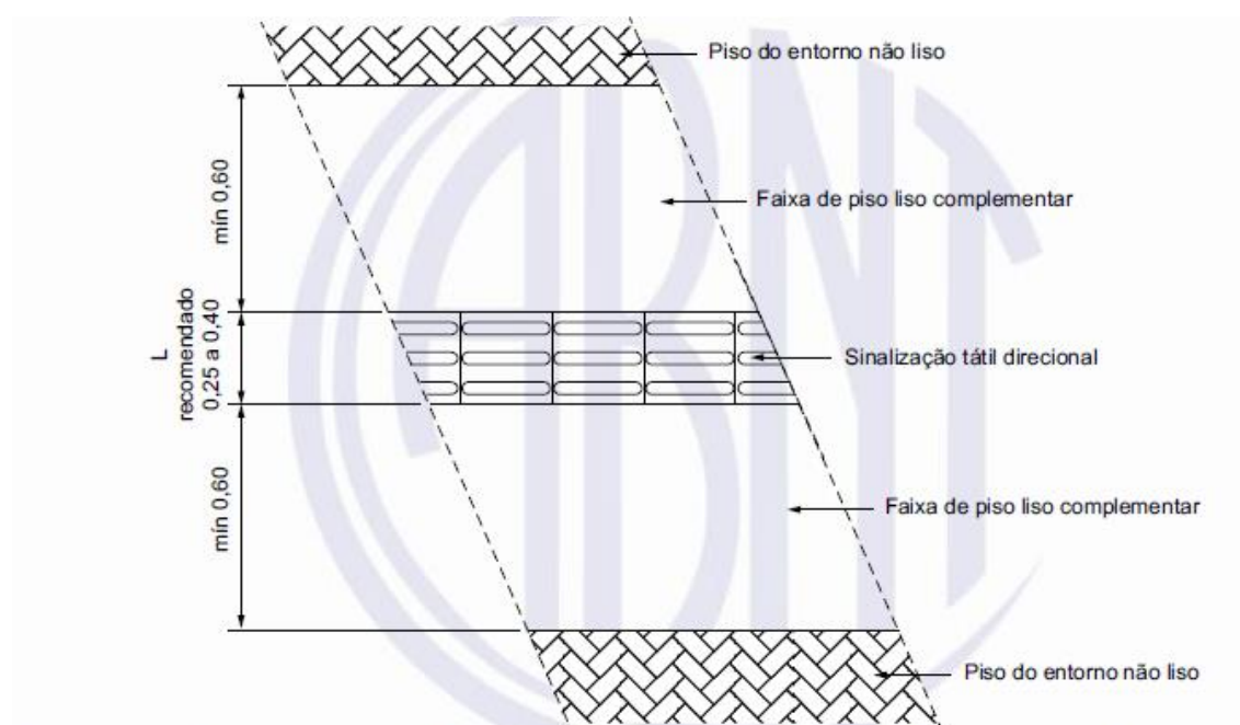
Figura 45 – Sinalização tátil direcional em piso com faixa lateral com piso liso complementar
