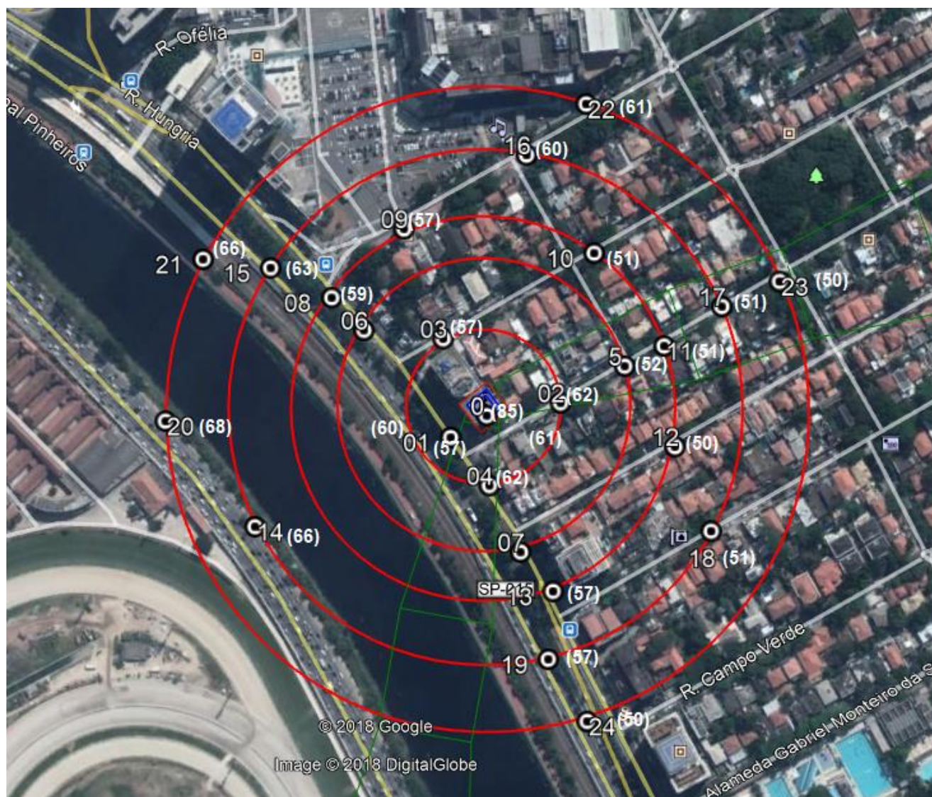
Fig. 06 – Levantamento do ruído produzido no meio ambiente pelo turno da manhã, com a operação do helicóptero na base do Heliporto QUADRA HUNGRIA, a 80% da potência.
