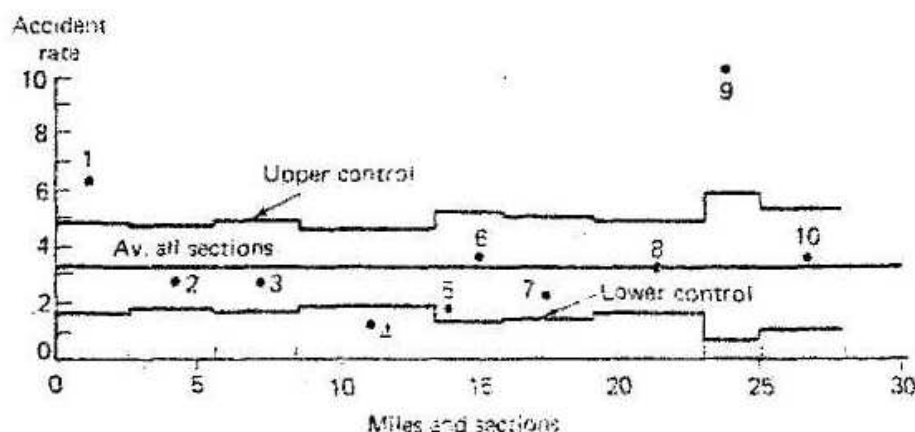
Figura 6. Representação das Seções Fonte: Baerwald (1976)
