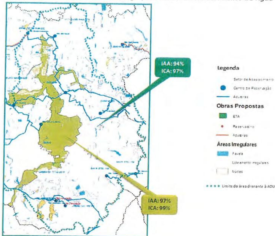
Figura 2.12 – Perímetro Jacu-Pêssego / Sistema de Abastecimento de Água
