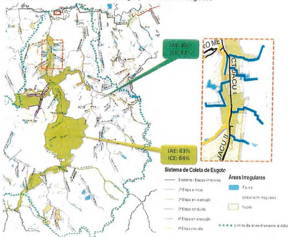
Figura 2.13 – Perímetro Jacu-Pêssego / Sistema de Esgotos
