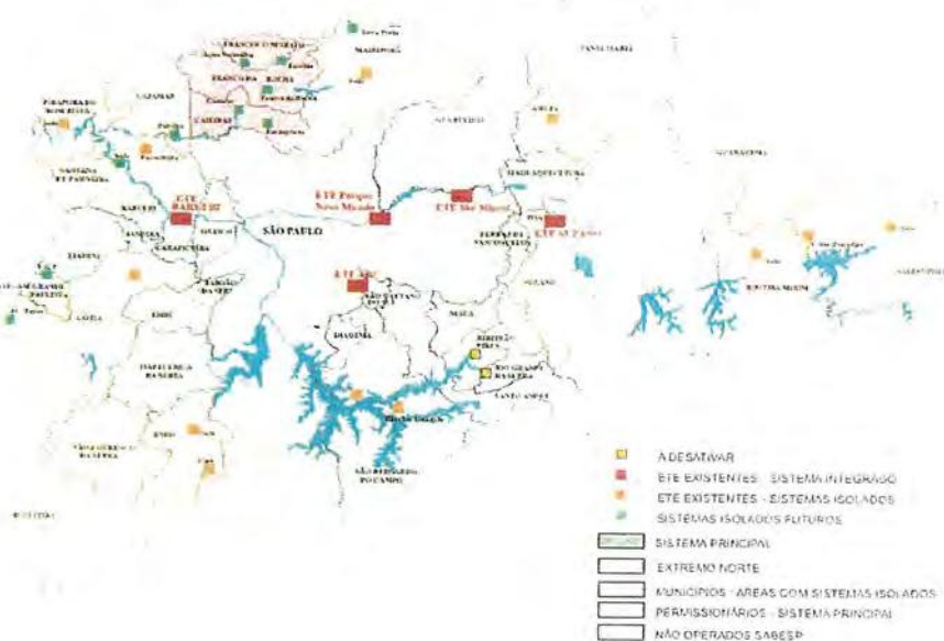
Figura 1.2 - Sistemas de Esgoto da Sabesp na RMSP
