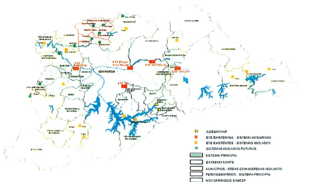
Figura 1.2 - Sistemas de Esgoto da Sabesp na RMSP
