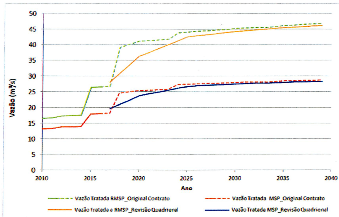
Gráfico 1.2 - Projeção da Vazão Tratada- Sistema Principal de Esgotos da RMSP
