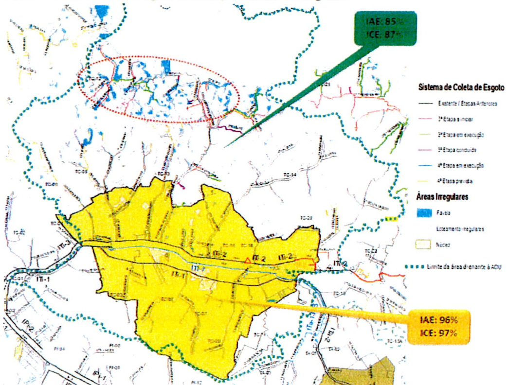
Figura 2.7 – Perímetro Água Branca / Sistema de Esgotos
