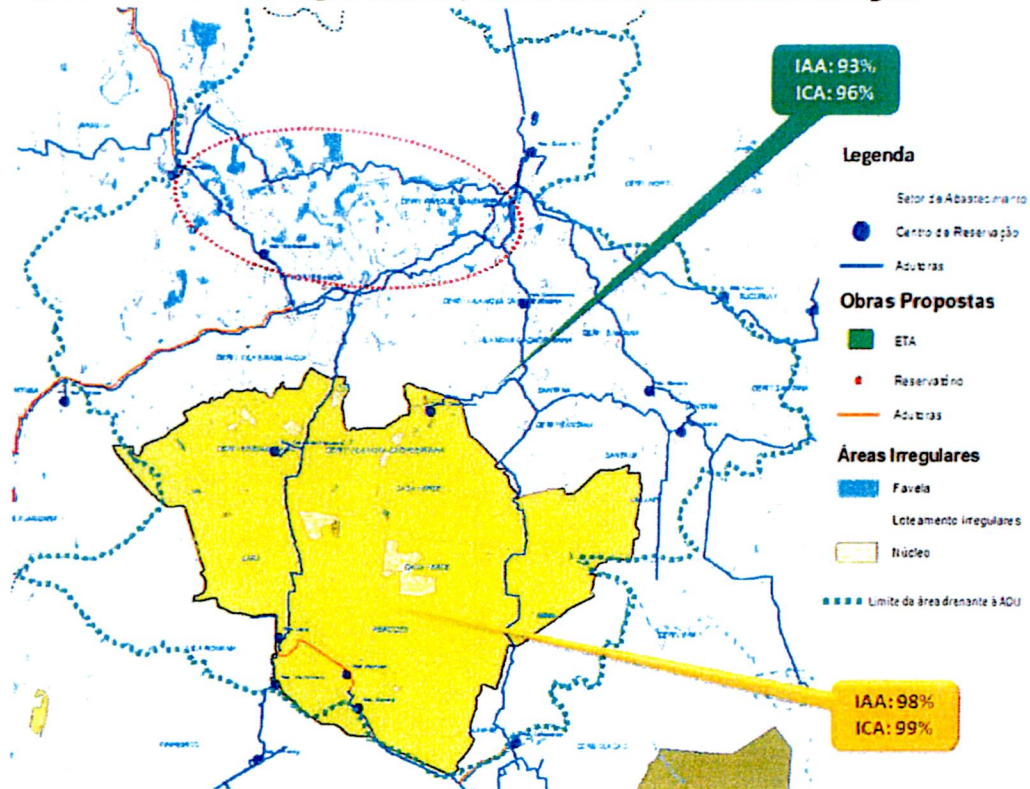
Figura 2.6 – Perímetro Água Branca / Sistema de Abastecimento de Água
