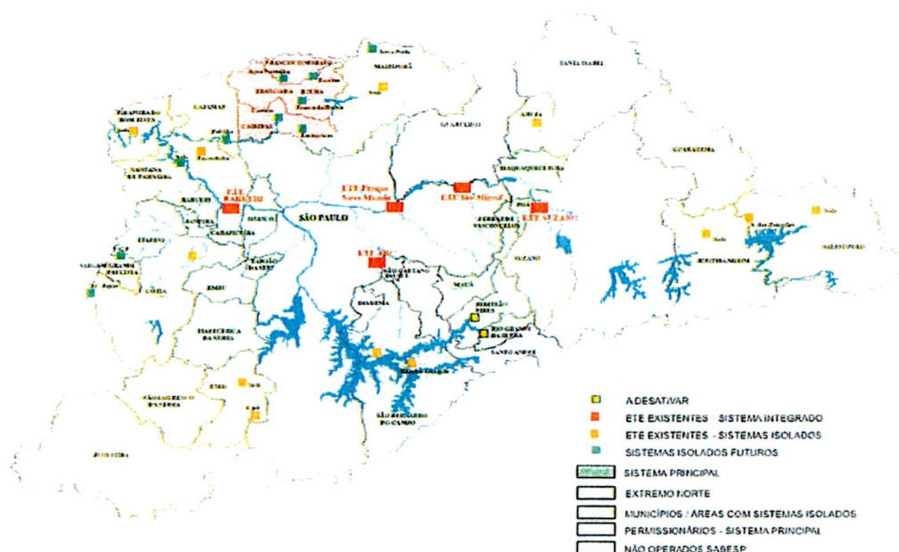
Figura 1.2 - Sistemas de Esgoto da Sabesp na RMSP
