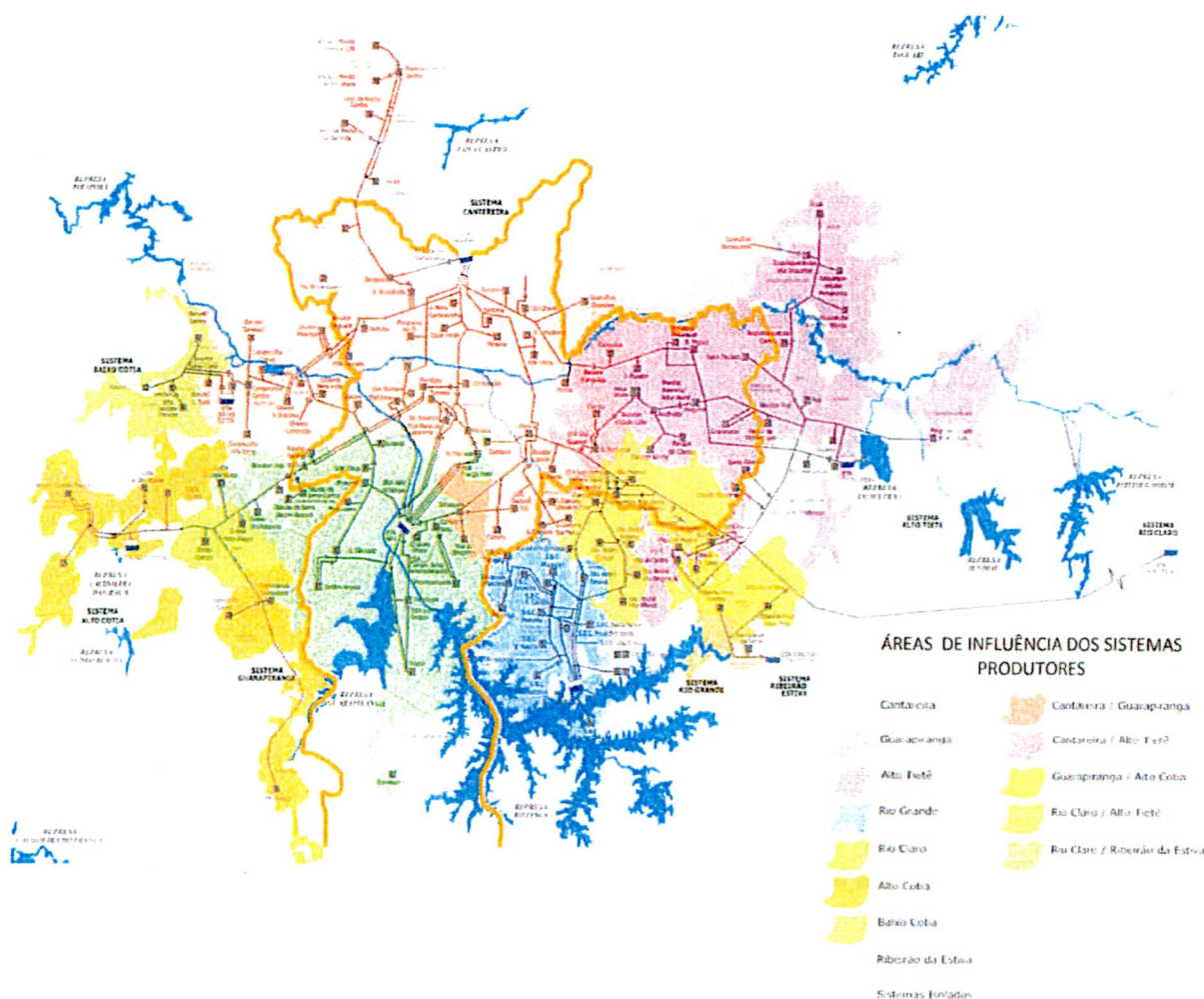
Figura 1.1 – Áreas de Influência dos Sistemas Produtores do SIM e Sistema Adutor Metropolitano – SAM
