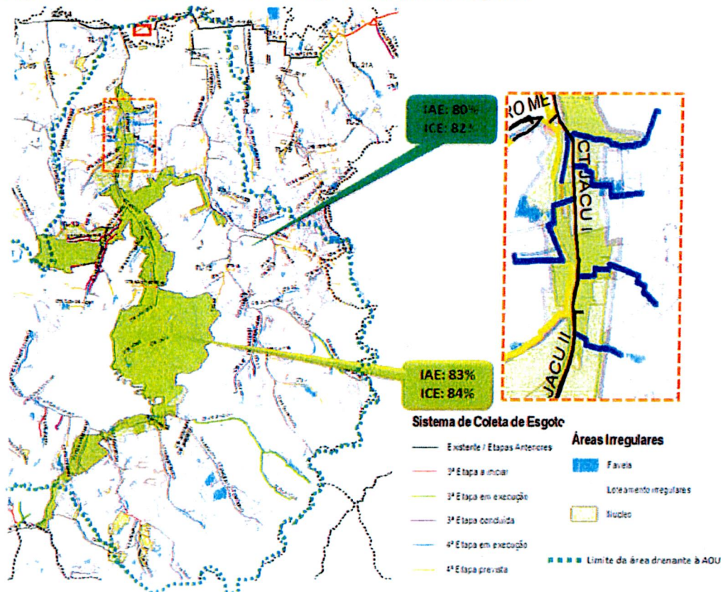
Figura 2.13 – Perímetro Jacu-Pêssego / Sistema de Esgotos
