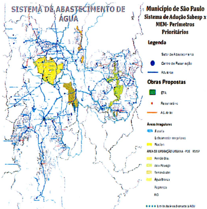
Figura 2.4 – Sistema de Abastecimento de Água / Perímetros Prioritários
