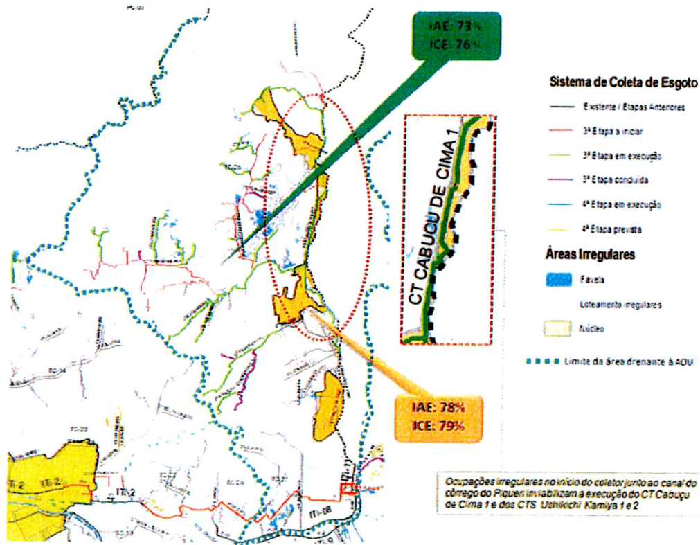
Figura 2.9 – Perímetro Fernão Dias / Sistema de Esgotos
