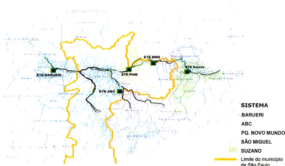
Figura 1.4 – Sistema Principal de Esgoto da RMSP - Áreas de Influência dos Sistemas de Tratamento – MSP
