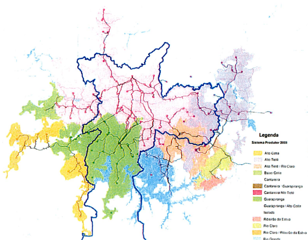
Figura 1.3 – Sistema Integrado de Metropolitano de Água - Áreas de Influência dos Sistemas Produtores - MSP
