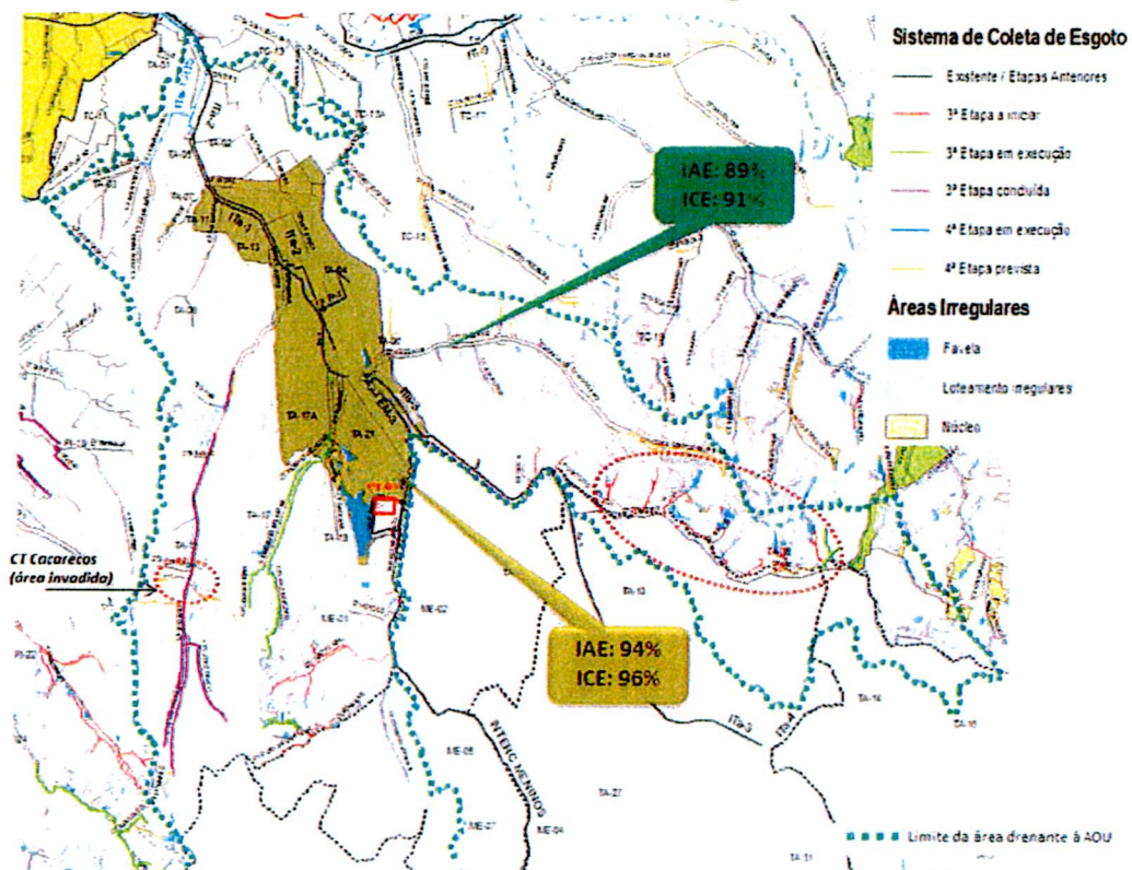
Figura 2.11 – Perímetro Tamanduateí / Sistema de Esgotos
