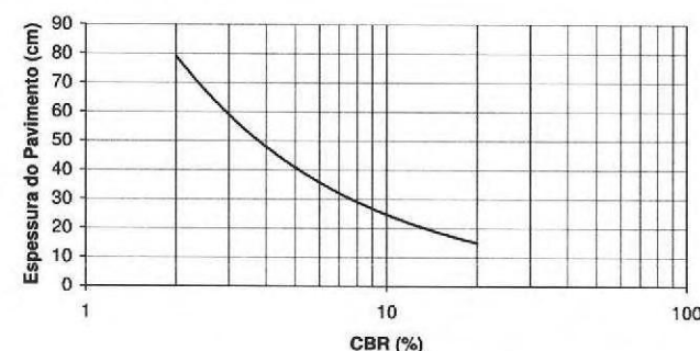
Figura 5.1 Ábaco de Dimensionamento
