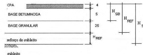
Figura 5.2 - Esquema Elucidativo
