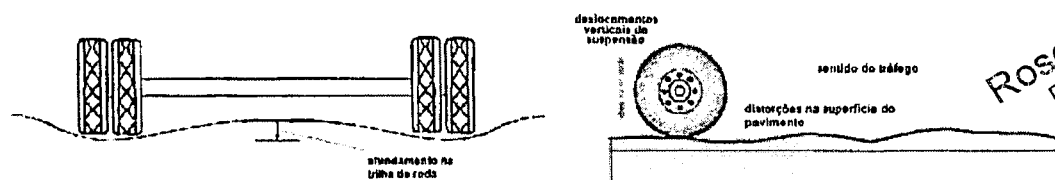
Figura 3 – Irregularidades (IRI) afetando custos de operação de veículos (fonte: Banco Mundial)
