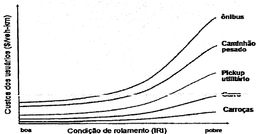
Figura 4 – Irregularidades superficiais nos pavimentos penalizam o rolamento dos veículos
