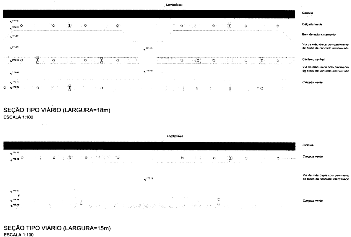
Figura 2 – Esquema ilustrativo da Av. Um.
