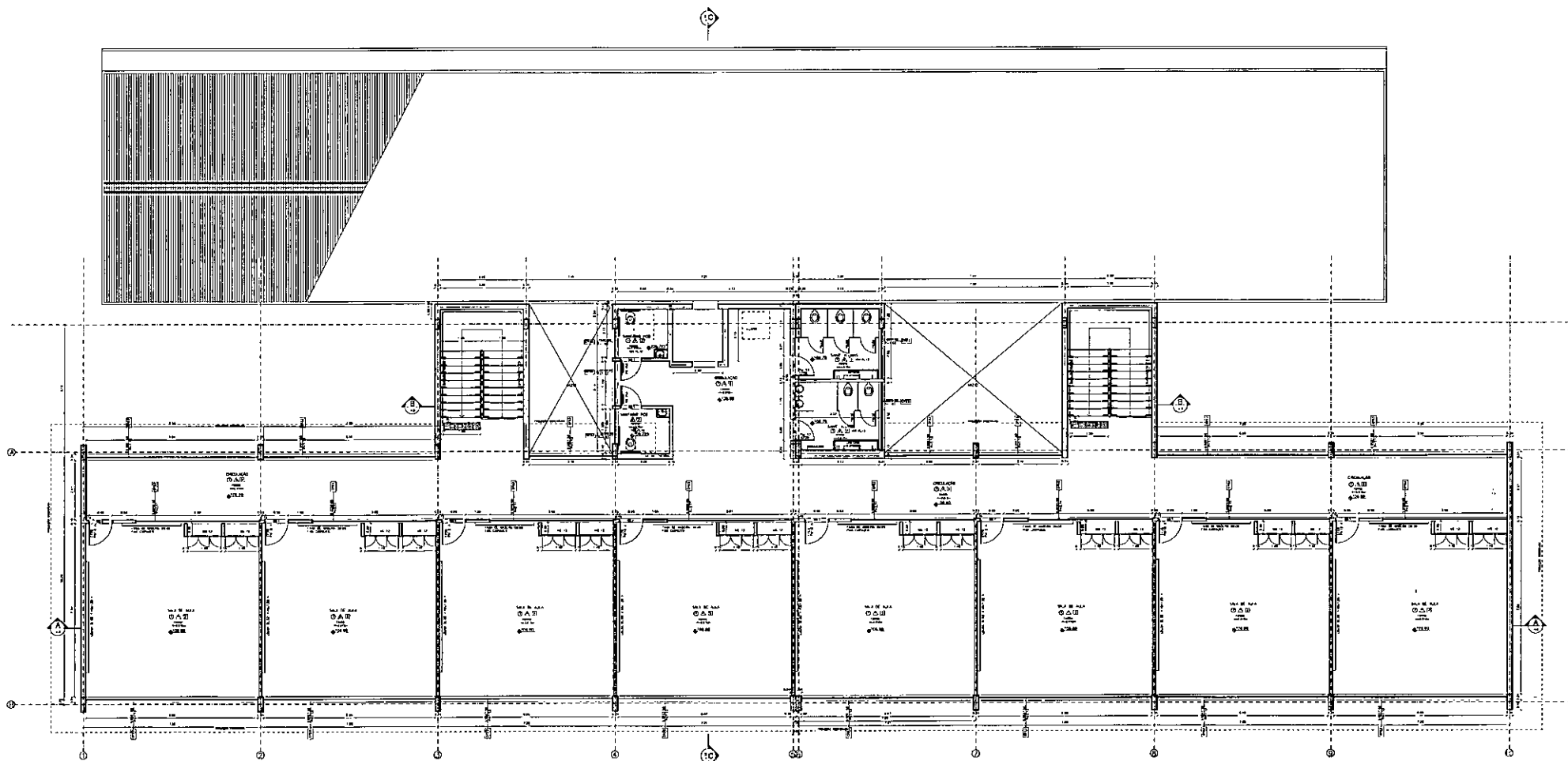
PLANTA PAVIMENTO SUPERIOR - CN 100 RD LSC 1:50
