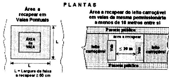
Figura 2 Demonstrativo da área a repor da capa Vala pontual ou longitudinal ou transversal
