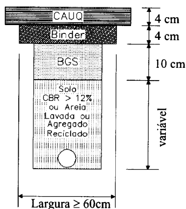
FIGURA 1A VALA Tráfego Leve Seção Tipo 1
