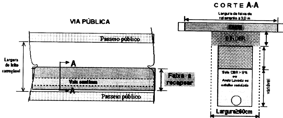
Figura 1 Demonstrativo da área a repor da capa Vala contínua
