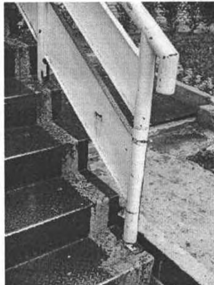
Fig. 62 – Detalhe corrimão
