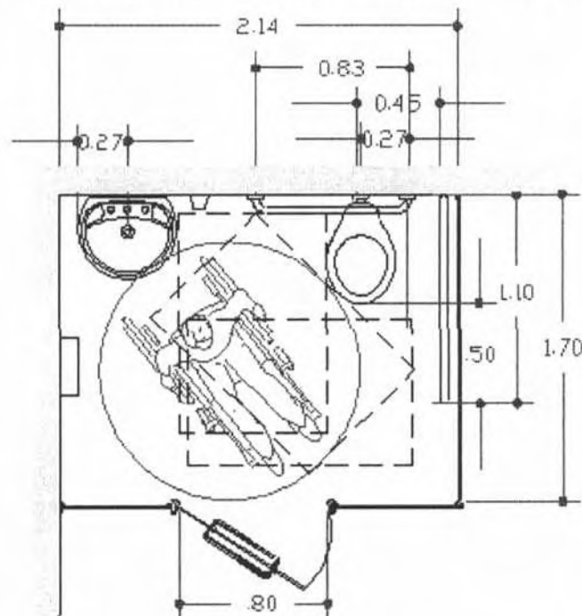
Boxe acessível - Sanitário Feminino
