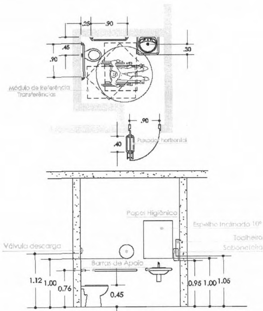
Fig. 6 – Vaso sanitário e barras de apoio.
