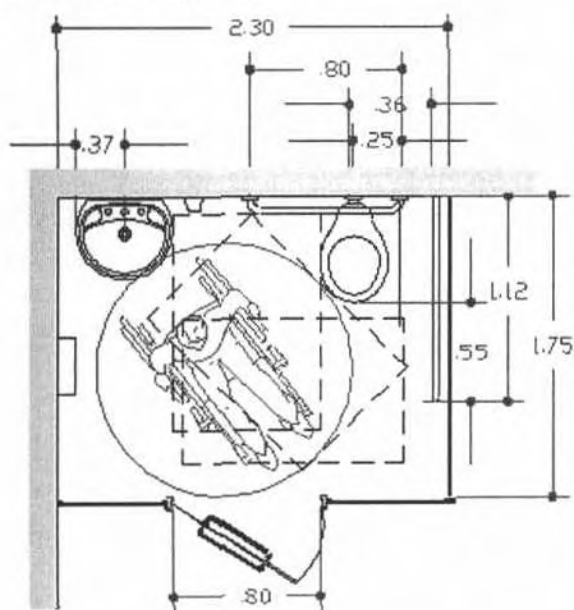
Boxe acessível - Sanitário Masculino
