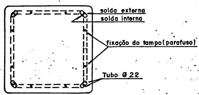
PLANTA
