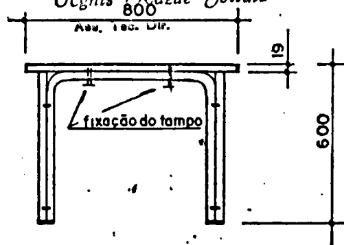
VISTA LATERAL
