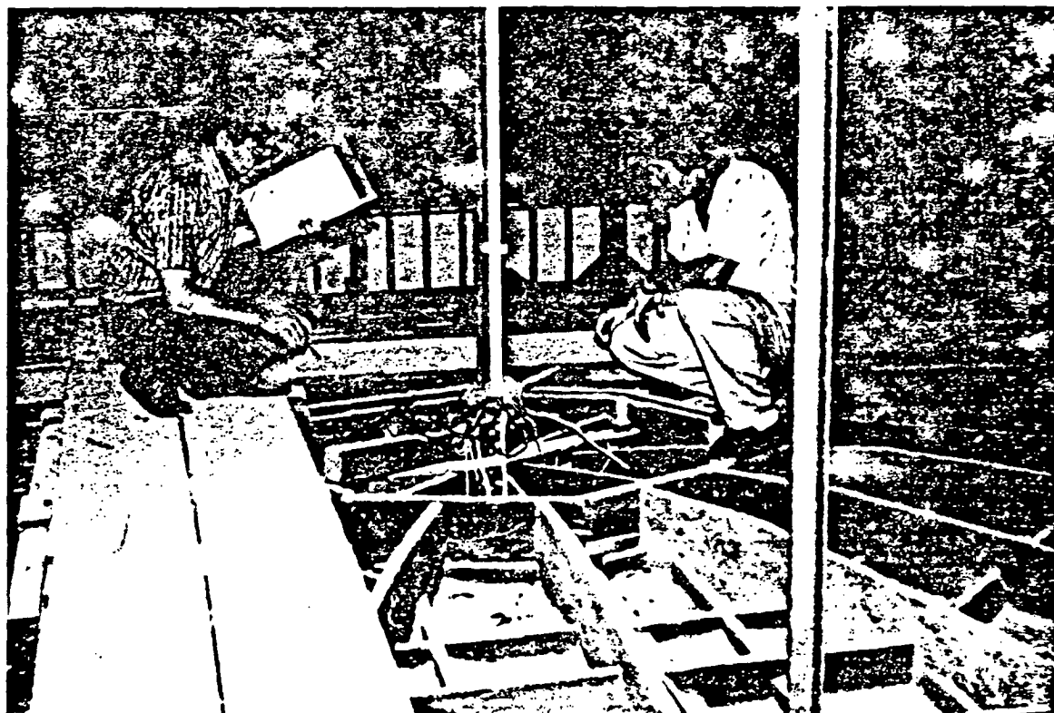
Fiação do lustre do Salão Azul, exposta sobre o madeiramento do forro.
